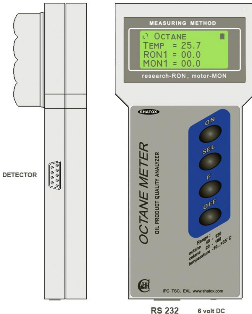
Рис.2. Внешний вид ОКТАНОМЕТРА (электронный блок)
