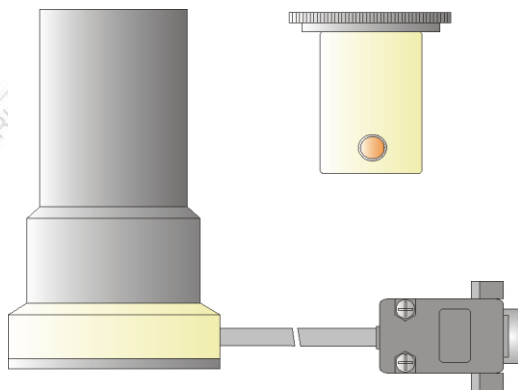
Рис.1. Датчик и имитатор пробы ОКТАНОМЕТРА
